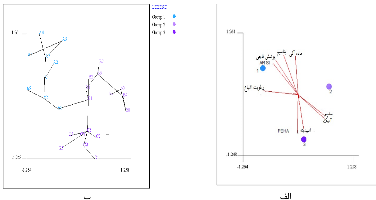
شکل ۳- الف - نتایج Principal axis correlation نشان داد که تعداد ۲ گونه گیاهی و ۵ پارامتر ادافیکی که به طور معنی داری با فضای رج بندی دو بعدی Multi Dimensional Scaling همبستگی داشته ( P < 0.05 ) و در سه گروه به شکل مرکزی نشان داده شده‌اند. شکل ب- تحلیل شبکه بندی را نشان می‌دهد (اندازه‌گیری پیوستگی با روش Bray & Curtis، تکنیک Flexible UPGMA، روش رج بندی SSH، در شکل شماره‌های ۱، ۲ و ۳ نشان‌دهنده مکان‌ها، بردارها معرف متغیرهای گیاهی و محیطی می‌باشند. علایم قرار داده شده برای گونه‌های گیاهی شامل Pe ha = Peganum harmala ، Arsi = Artemisia sieberi است.
